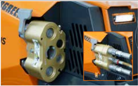
Acoplamientos rápidos hidráulicos CE3N Engates rápidos hidráulicos CE3N
